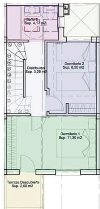
PRIMERA PLANTA FIRST FLOOR
